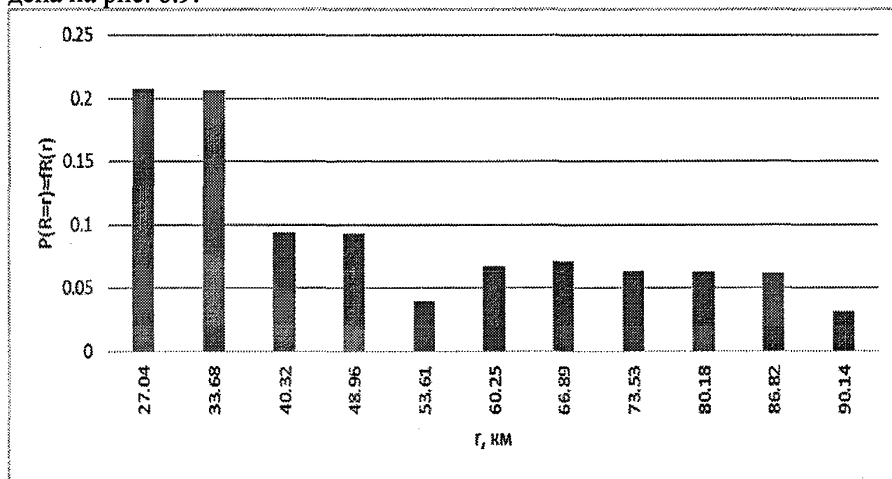
Рис. 6.9. Аппроксимация функции f_R(r) для источника № 1
