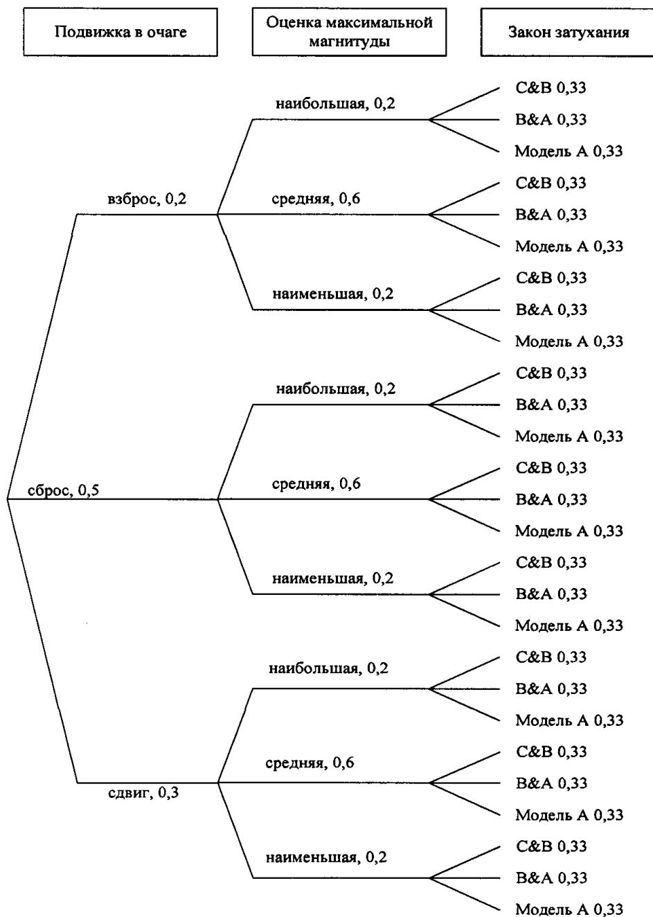
Рис. 6.2. Фрагмент логического дерева анализа неопределенности
