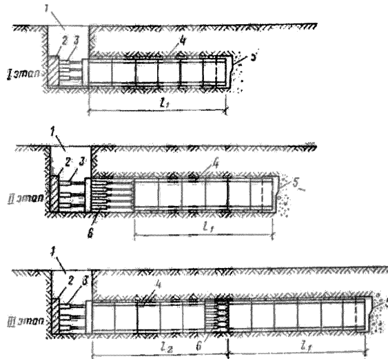
1 – стартовый котлован; 2 – упор; 3 – домкратная установка в стартовом котловане; 5 – ножевая секция; 6 – промежуточная домкратная установка.
