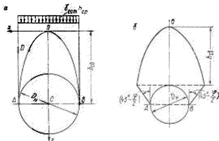
а) – опирание свода на уровне центра трубы; б) – опирание свода на уровне верхней образующей трубы
