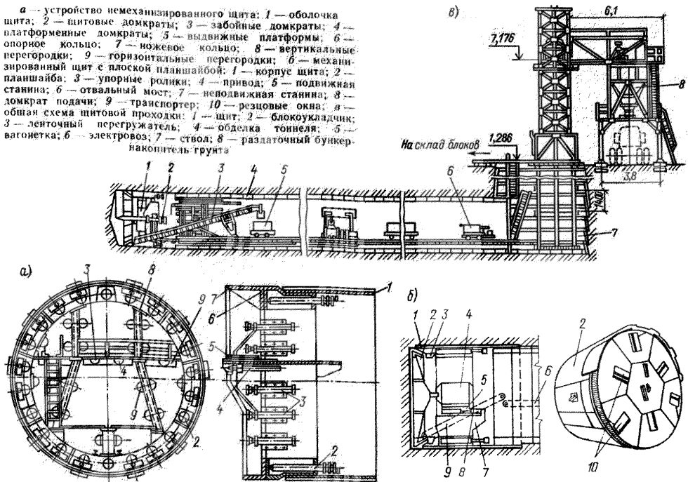
а) немеханизированный щит; б) механизированный щит; в) общая схема щитовой проходки
