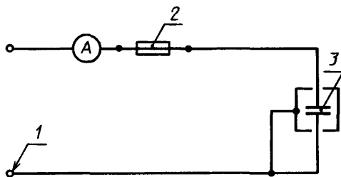
1 — источник переменного тока; 2 — предохранитель; 3 — конденсатор
