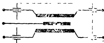
Рис. 4.4 Многосекционный проходной конденсатор
