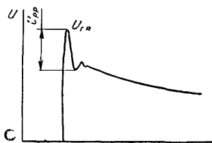
Рис. 6 Форма импульса
