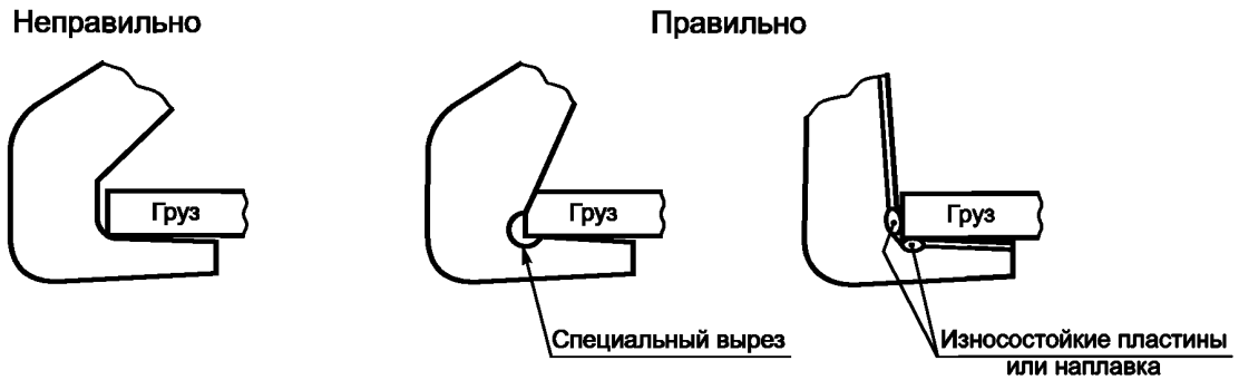
Рисунок 4 — Конструкция захватов ГЗП
