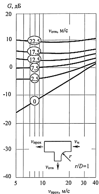
б) тройник с закругленными кромками
