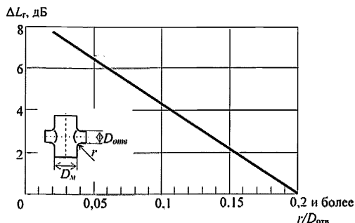
Рисунок 6.5 – Поправка \Delta L_g , учитывающая влияние радиуса закругления ответвления на шумообразование
