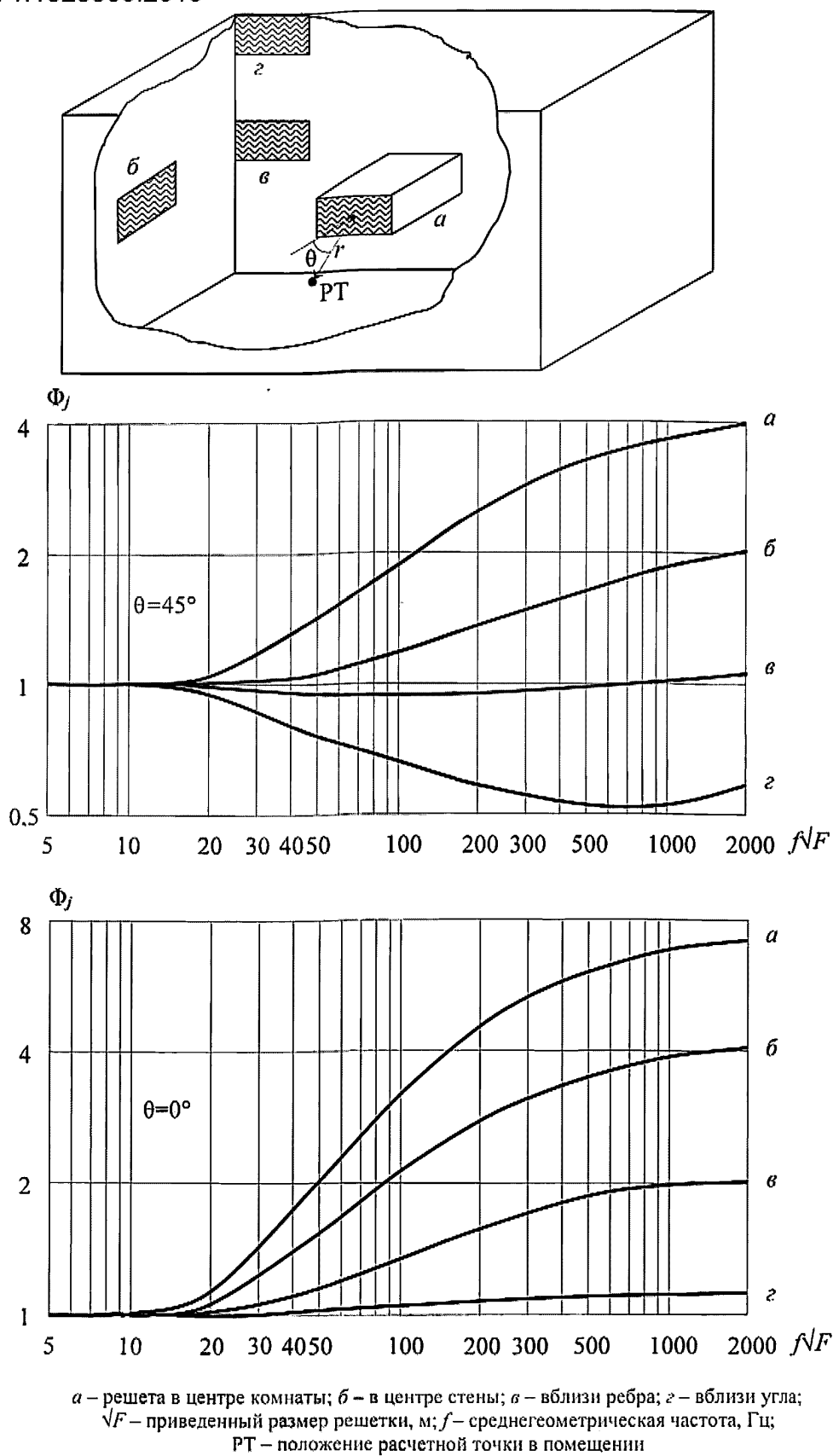
Рисунок 8.1 – Фактор направленности \Phi_j
