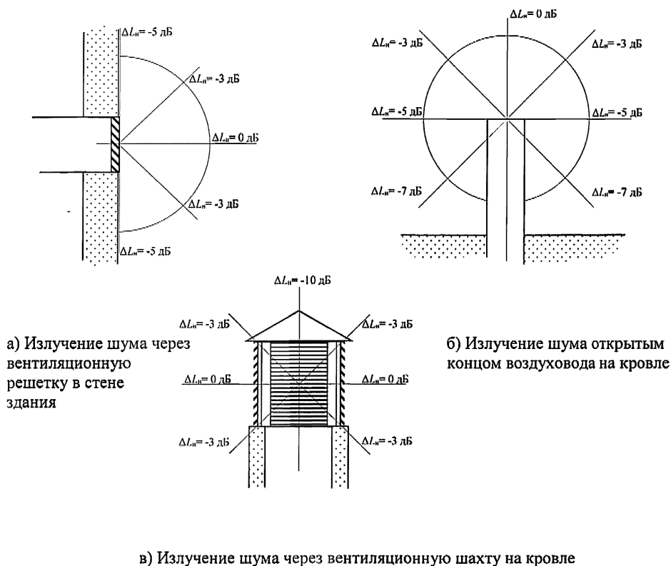
Рисунок 8.3 – Показатель направленности излучения шума через отверстия вентиляционных решеток, воздухопроводов, шахт и подобных элементов
