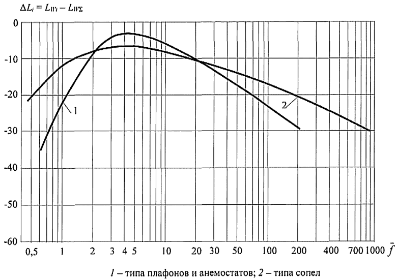
Рисунок 6.13 – Безразмерные частотные характеристики воздухораспределителей
