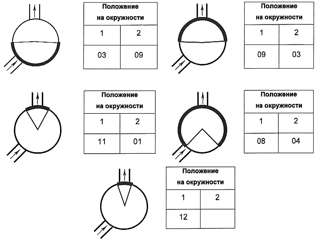
Рисунок 3 — Примеры определения координат объекта на окружности
