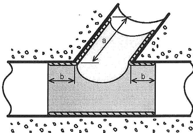
Рисунок 20 — Т-образная манжета
