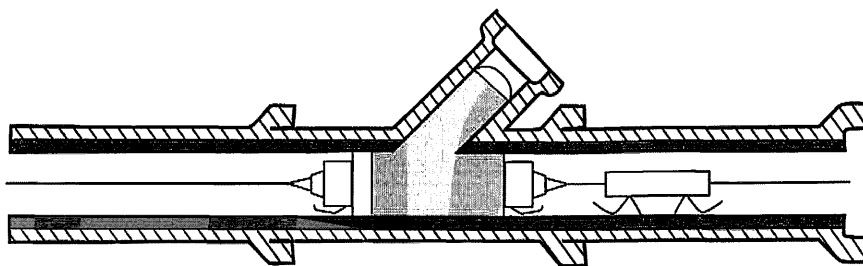
Этап 2. Позиционирование манжеты и ее затверждение.
