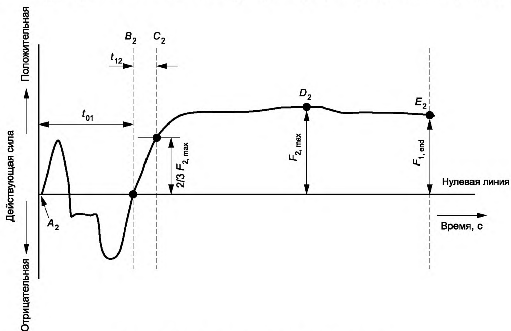
Рисунок Е.3 — Сила смачивания припойной пасты
