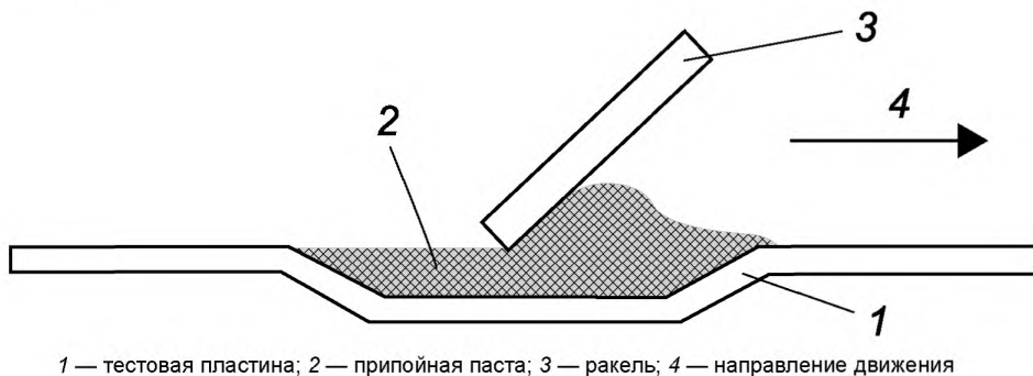
Рисунок 4 — Пример применения припойной пасты к тестовой пластине
