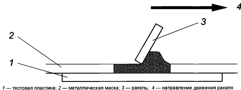
Рисунок 11 — Пример нанесения припойной пасты на тестовую пластину
