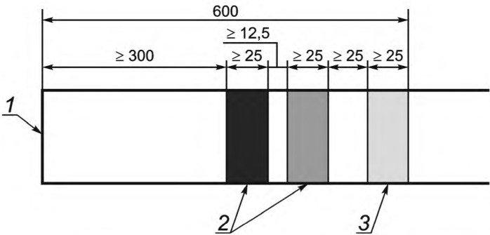
1 — торец изделия; 2 — полосы, указывающие на марку материала; 3 — полоса, указывающая на группу прочности
