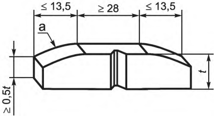
a Кривизна, обусловленная наружным диаметром изделия.
