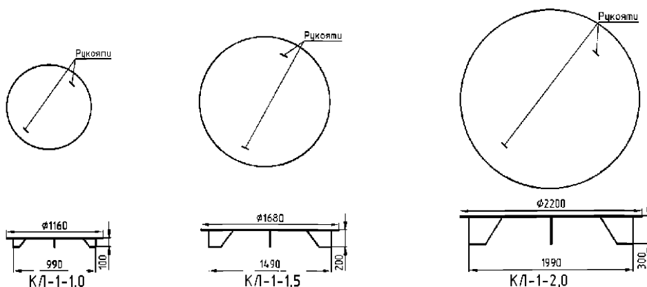
Рис. 1. Крышки КЛ-1.
