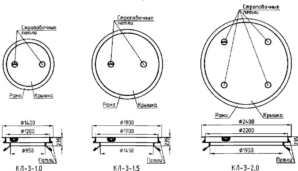
Рис. 3. Крышки КЛ-3.
