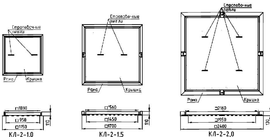
Рис. 2. Крышки КЛ-2.
