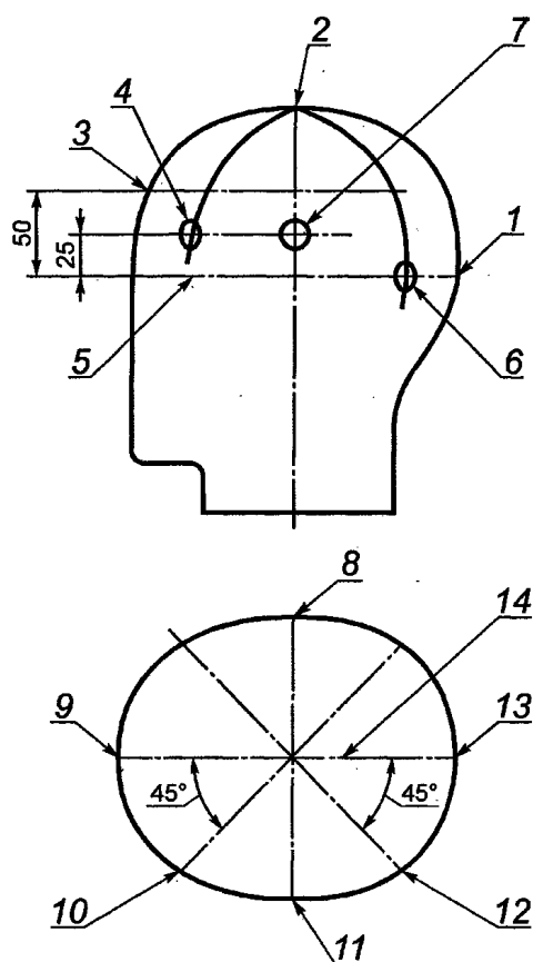
Рисунок 1 — Ориентирующие плоскости
