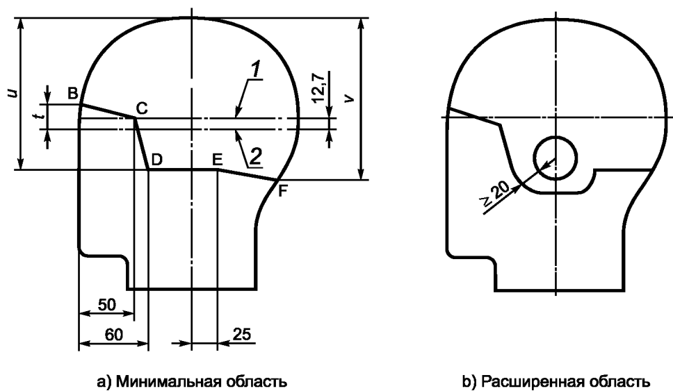
1 — контрольная плоскость; 2 — основная плоскость
