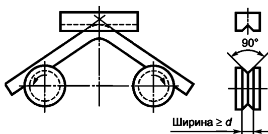
Рисунок Б.2 — Схема устройства для разгиба
