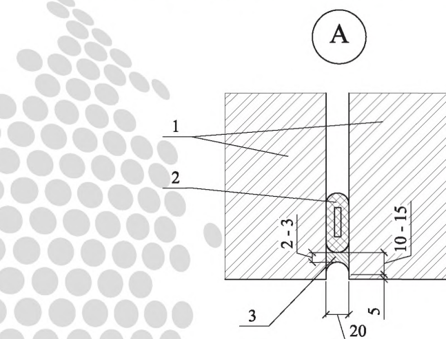
Рисунок А.2.10 - Деформационный шов в защитно-декоративной кладке (Узел 4)
