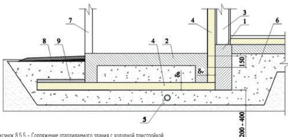
Рисунок 8.5.5 – Сопряжение отапливаемого здания с холодной пристройкой
