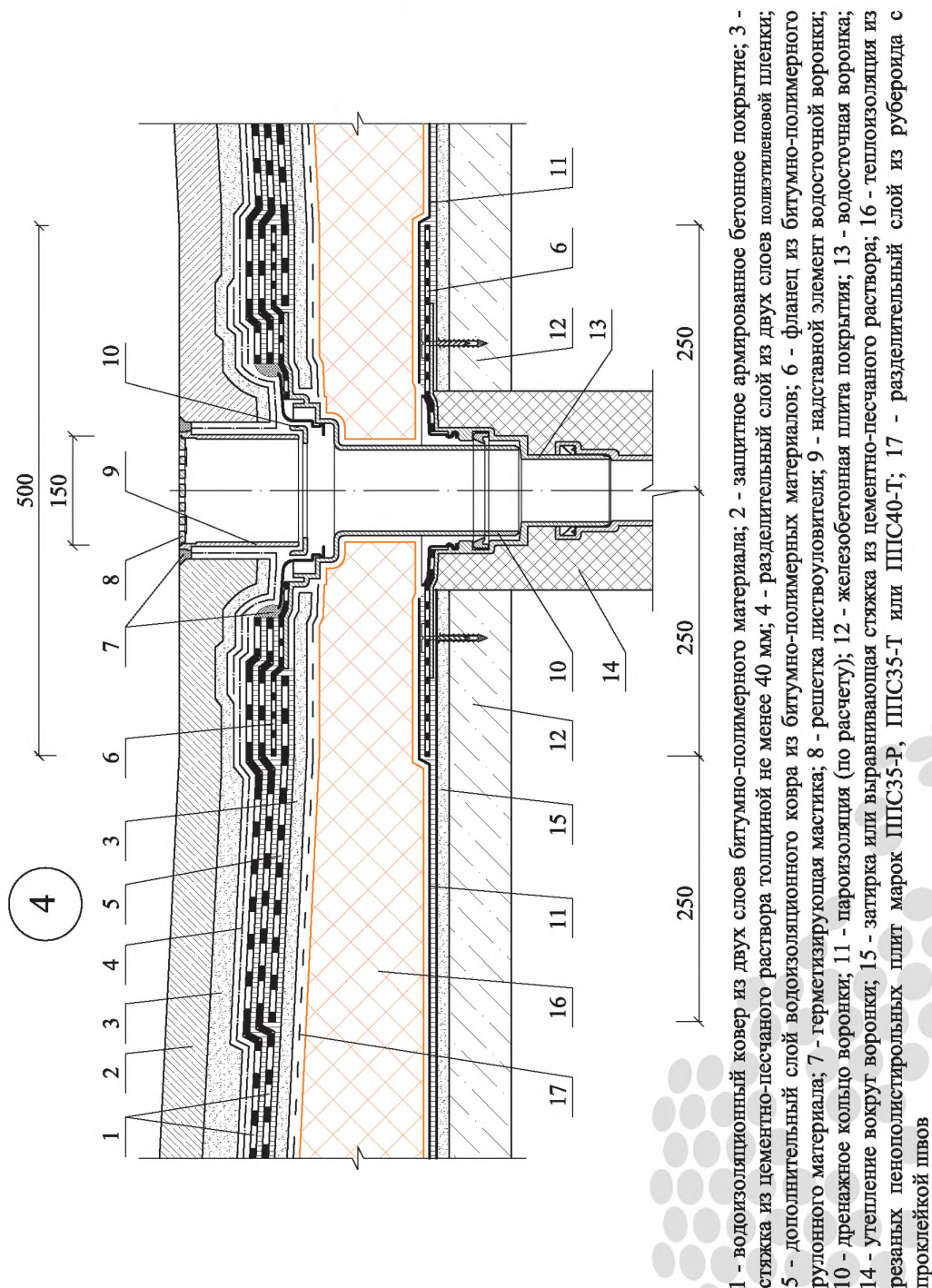
Рисунок А.6.10 - Присоединение к воронке (Узел 4)
