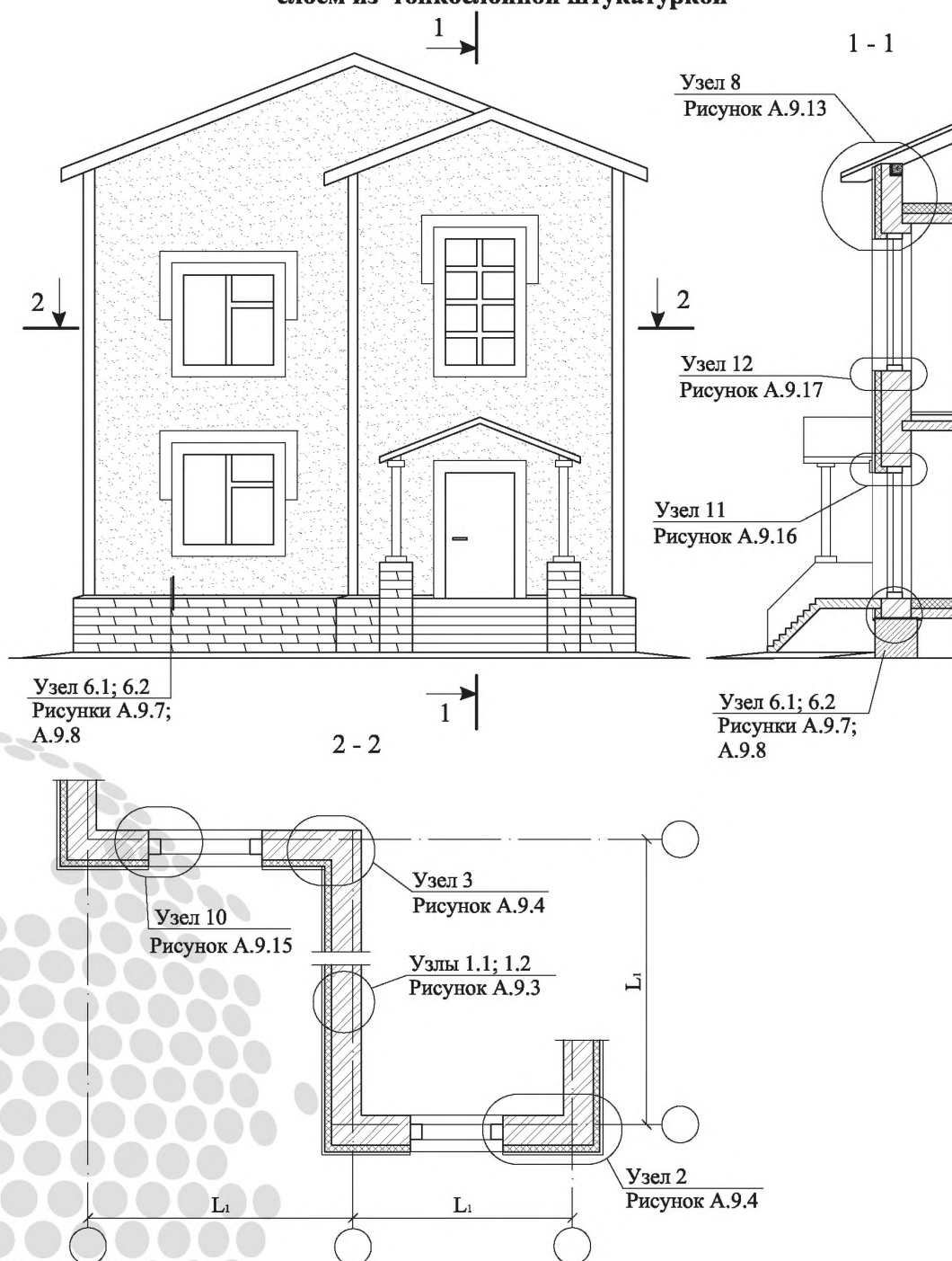
Рисунок А.9.1 - Фасад здания, разрезы 1-1 и 2-2
