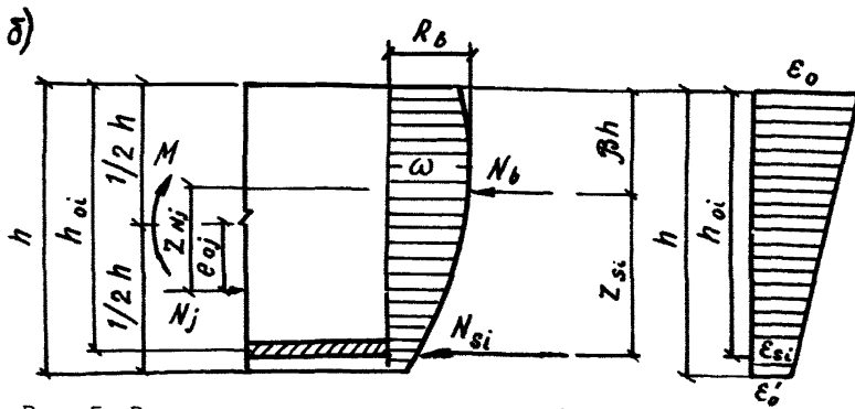
Рис. 5. Расчетная схема внутренних усилий и распределения деформаций в сечении элемента
