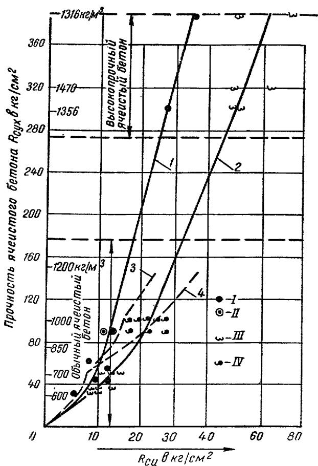
Рис. 23. Зависимость R_{сж} от R_{сж}
