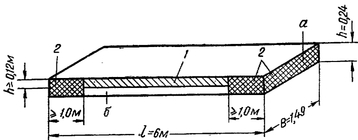
Рис. 8. Зоны в газосиликатных плитах марок ГКП, в которых недопустимы усадочные технологические трещины \alpha — торцовая грань плиты; b — продольная грань плиты; 1 — недопустимы горизонтальные трещины; 2 — недопустимы горизонтальные и косые трещины
