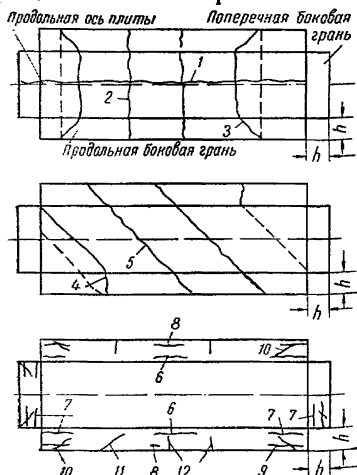
Рис. 7. Возможные варианты образования усадочных трещин в плитах марок ГКП
