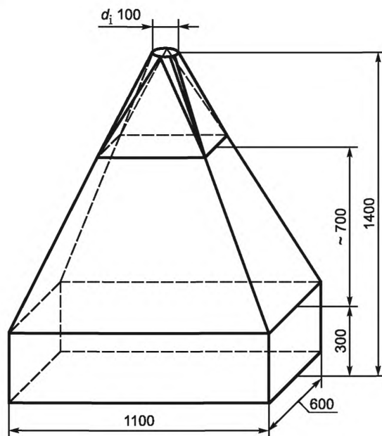
Рисунок 25 — Испытательный кожух
