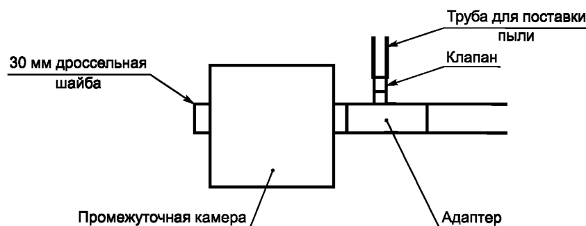
Рисунок 10 — Подсоединение трубки к отверстию
