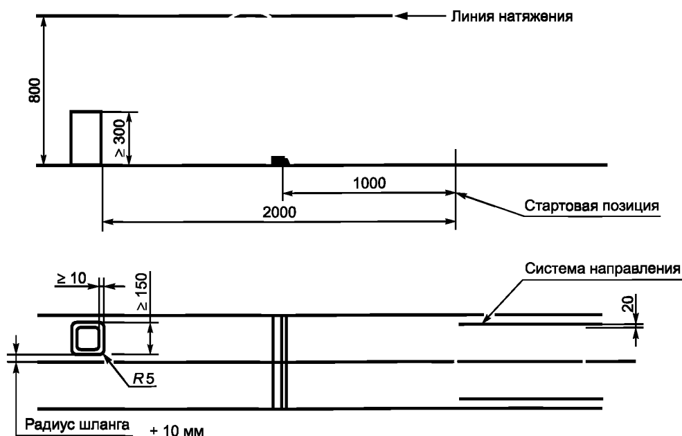
Рисунок 15 — Методы испытания ударом
