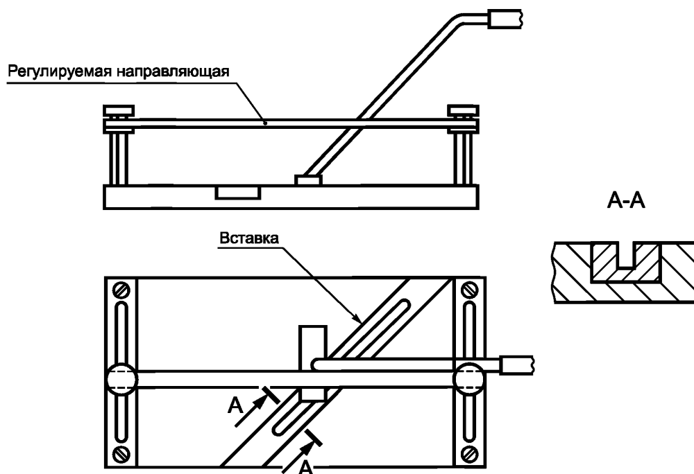
Рисунок 18 — Испытательная пластина со щелью
