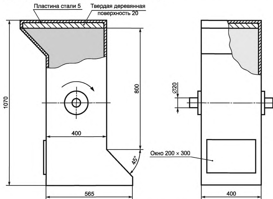
Рисунок 28 — Барабан для испытания на воздействие
