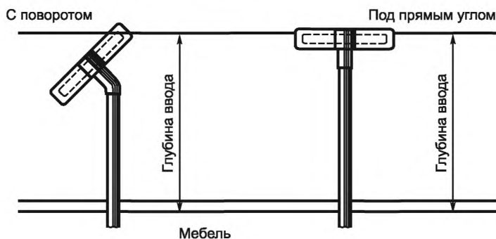
Рисунок 12 — Глубина ввода
