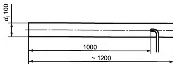
Рисунок 27 — Выхлопной канал с выборкой для исследования
