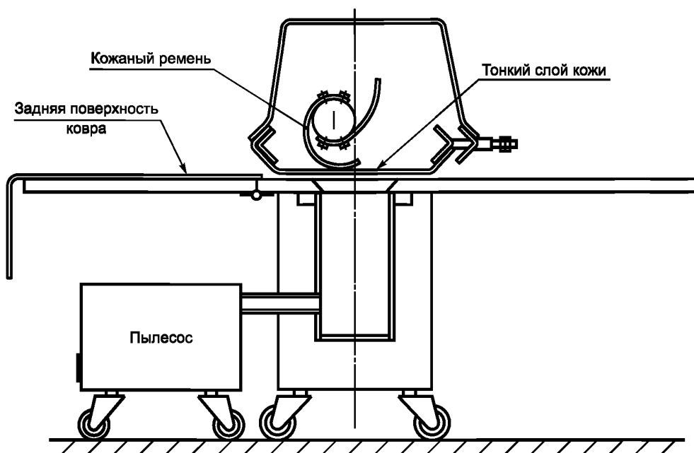
Рисунок 19 — Машина для выбивания ковра
