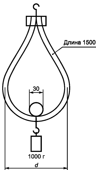
Рисунок 16 — Подготовка шлангов для испытания на гибкость
