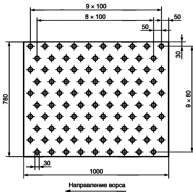
Рисунок 3 — Трафарет для распределения волокон по испытательным коврам
