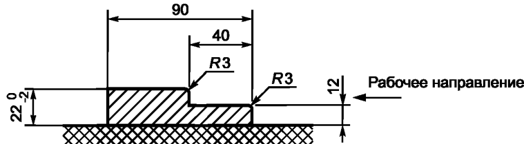
Рисунок 14 — Профиль порога
