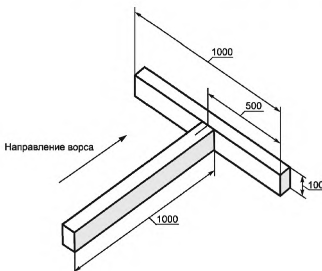
Рисунок 1 — Т-образная конструкция
