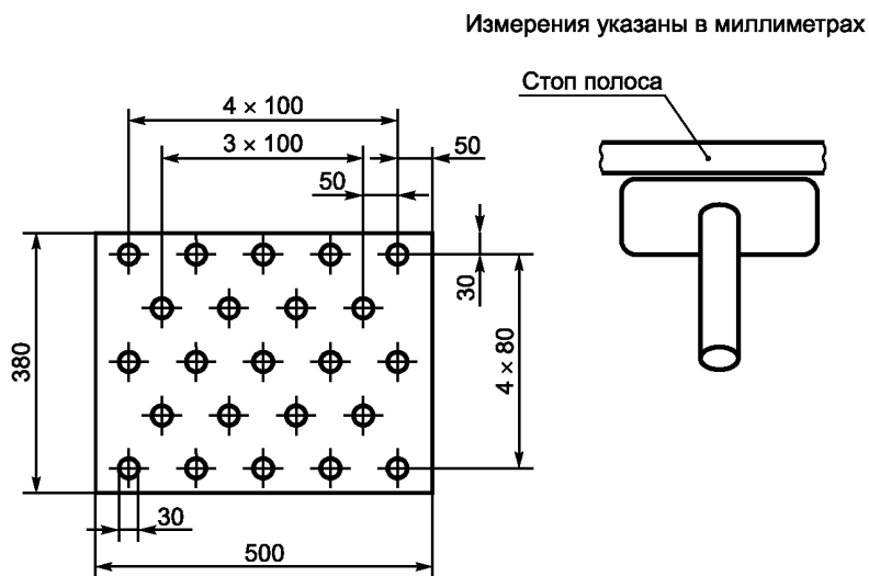
Рисунок 6 — Трафарет для распределения волокон на обивке
