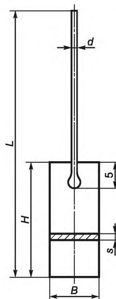
Рисунок А.3.12 — Пластиновый электрод из платины (Изделие № 318)
