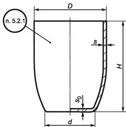
Рисунок А.1.3 — Высокий тигель из серебра (Изделие № 102)
