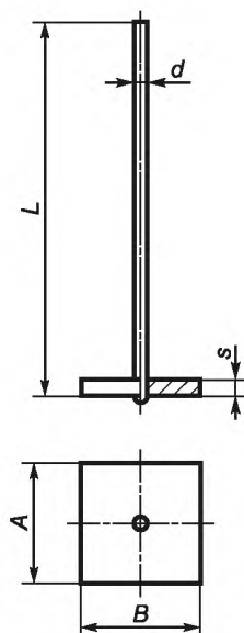
Рисунок А.3.13 — Пластиновый электрод из платины (Изделие № 319)
