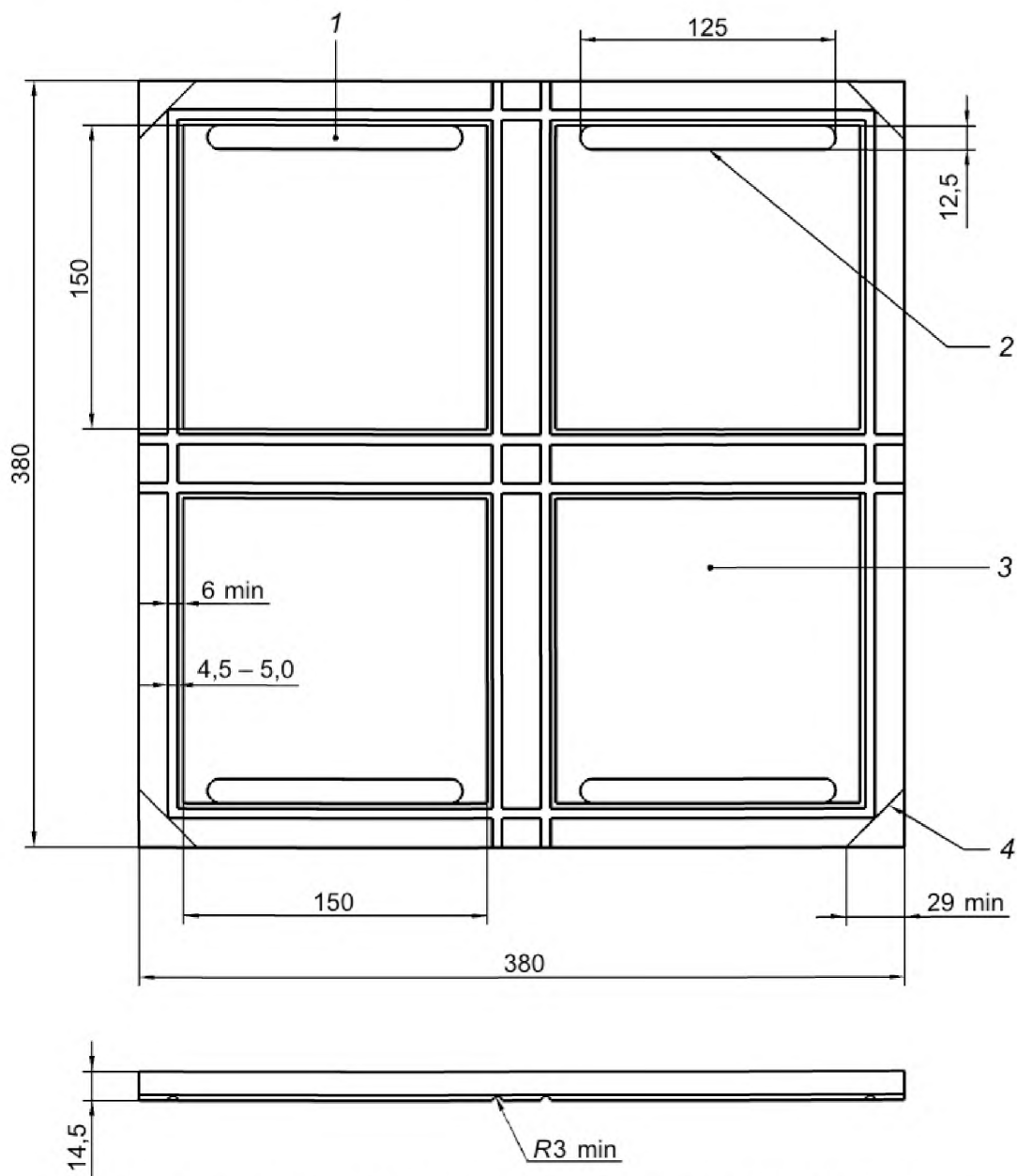
Рисунок 1 — Четырехгнездная пресс-форма
