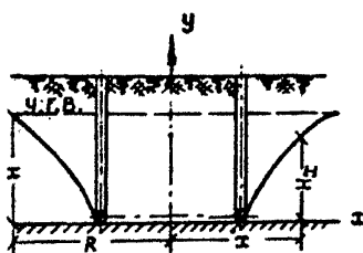
Рис. 27. Систематический дренаж
