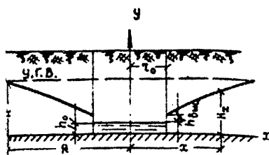
Рис. 29. Пластовый дренаж.
