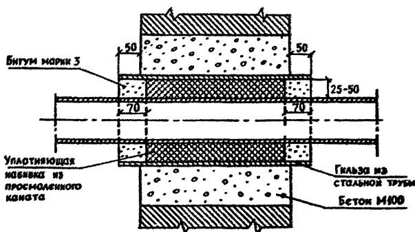
Рис. I. Заделка отверстий для пропуска трубопроводов в стенах подвалов.
