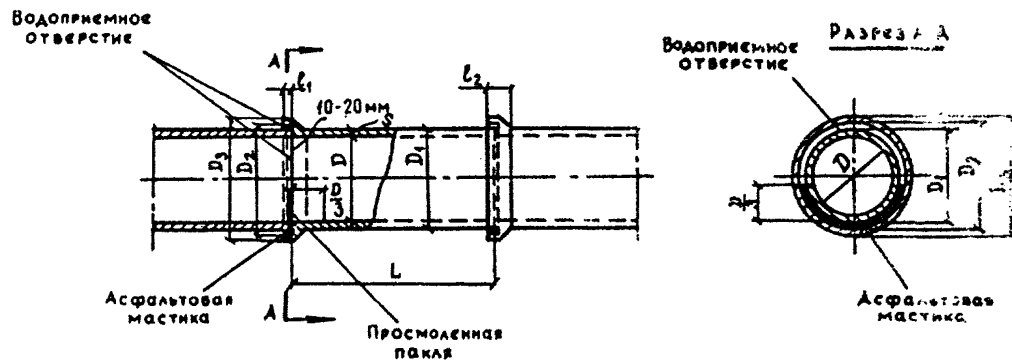
Рис. I8 Керамические трубы. Заделка отрыва.
