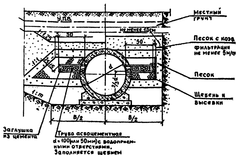
Рис. 14. Дренажное устройство на водостоке.
