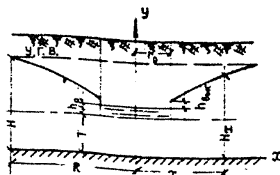
Рис. 29. Пластовый дренаж.
