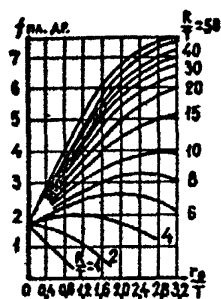
Рис. 85. График функции f пл. др.
