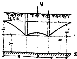
Рис. 27. Систематический дренаж
