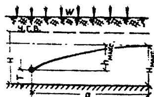
Рис. 27. Систематический дренаж
