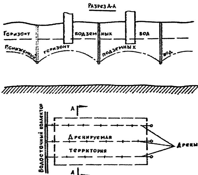
Рис. 7 Схема систематического дренажа.
