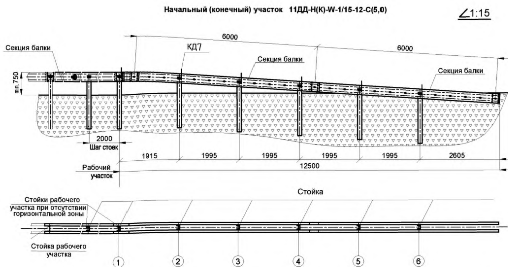
Рисунок 8 – Схема и состав начального (конечного) участка с уклоном 1:10
