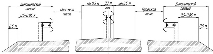
Рисунок 13 – Установка барьерного дорожного ограждения с отделяющейся балкой.
