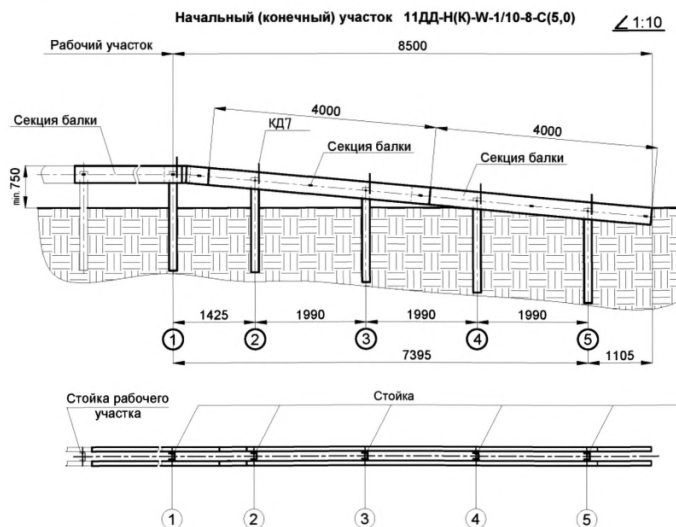
Рисунок 7 – Схема и состав начального (конечного) участка с уклоном 1:15
