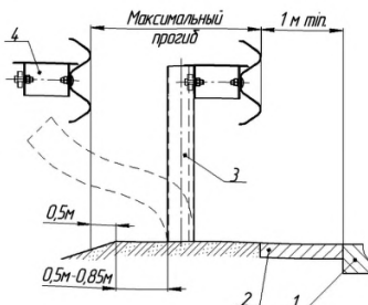
Рисунок 14 – Максимальный прогиб одностороннего барьерного ограждения
