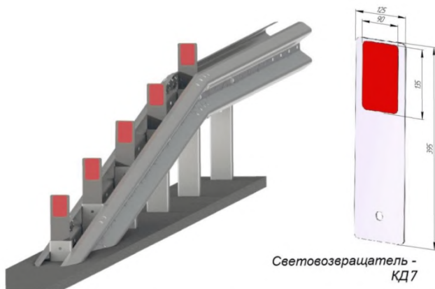
Рисунок 9 – Общий вид начального (конечного) участка со световозвращателем типа КД7
