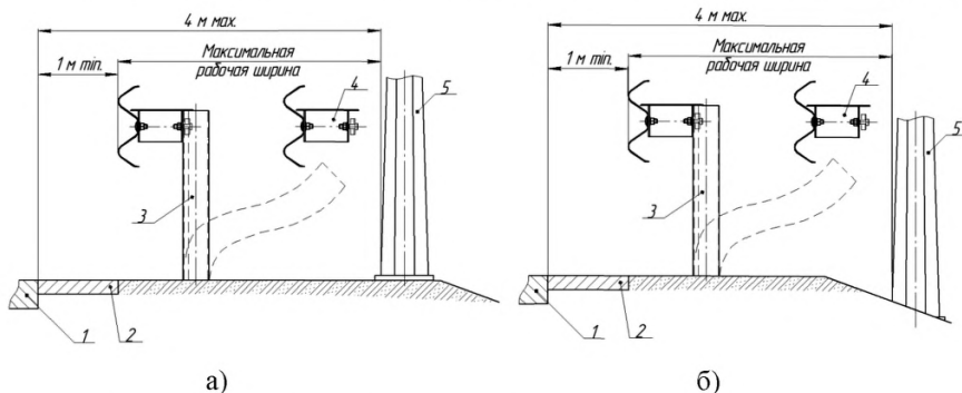
Рисунок 15 – Максимальная рабочая ширина до массивного препятствия :
