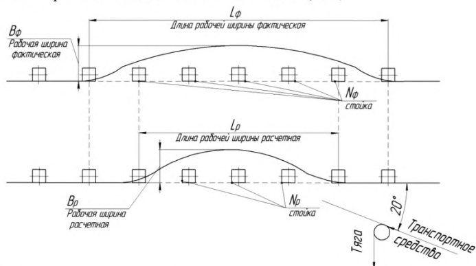
Рисунок 5 – Работа барьерного дорожного ограждения с отделяющей балкой устанавливаемой на обочине проезжей части при наезде ТС с большей энергией
