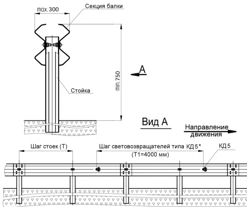
Рисунок 4а – Схема конструкции барьерного дорожного ограждения с отделяющей балкой устанавливаемой на оси проезжей части.
