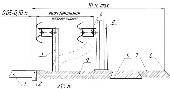
Рисунок 16 – Максимальная рабочая ширина до массивного препятствия
