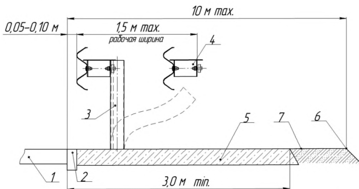
Рисунок 17 – Максимальная рабочая ширина барьерного ограждения с отделяющей балкой устанавливаемого на тротуаре.
