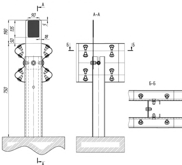
Рисунок 12 – Основные параметры установки световозвращателя КД7 на барьерном дорожном ограждении с отделяющей балкой.
