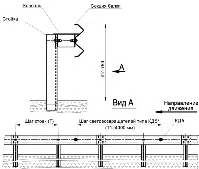
Рисунок 4б – Схема конструкции барьерного дорожного ограждения с отделяющей балкой устанавливаемой на обочине проезжей части.
