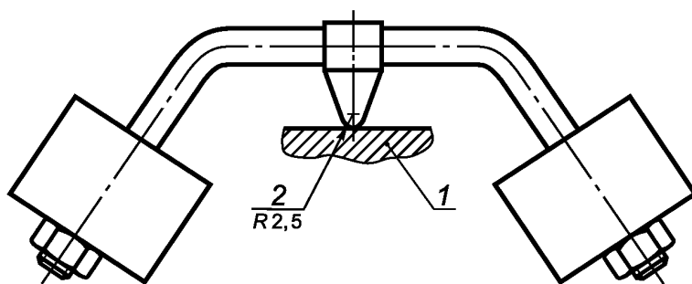
1 — образец; 2 — сфера
