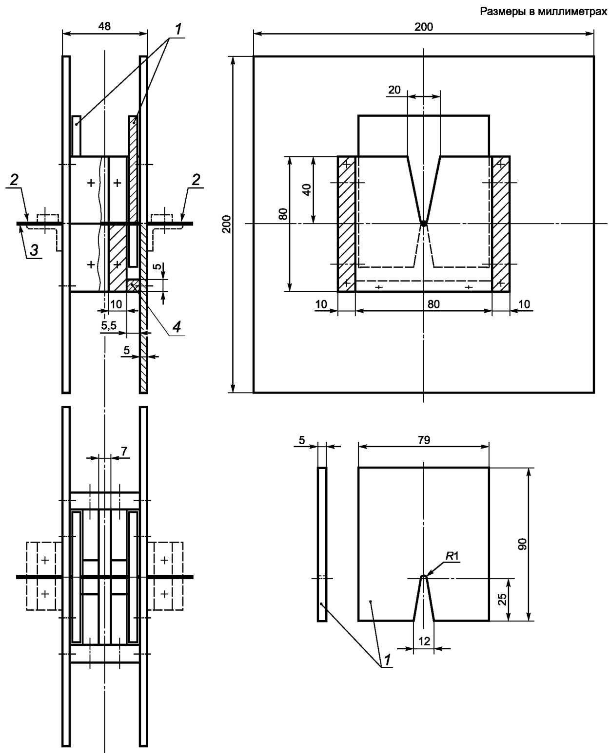
Рисунок ИЕ.1 — Испытательное устройство для проверки устойчивости УЗДП к минимальным значениям I^2t и I_p
