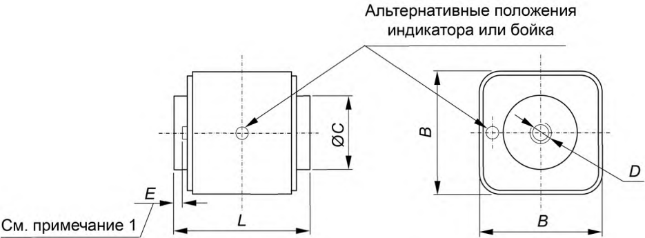
Корпуса размеров 00, 0, 1, 2 и 3
