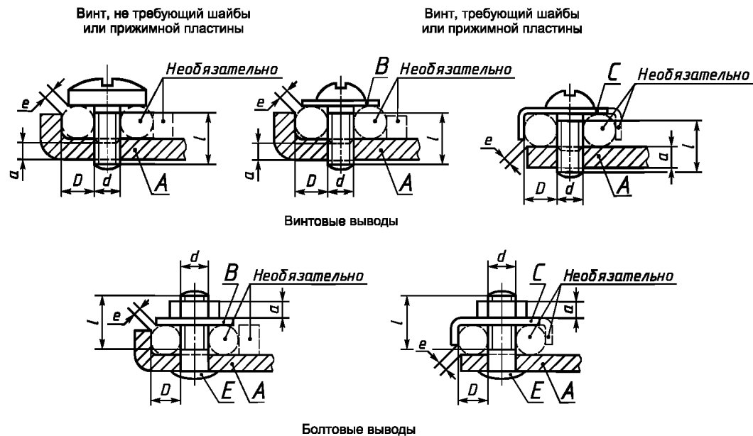
A — фиксирующая часть; B — шайба или прижимная пластина; C — приспособление, препятствующее выскальзыванию провода; E — болт
