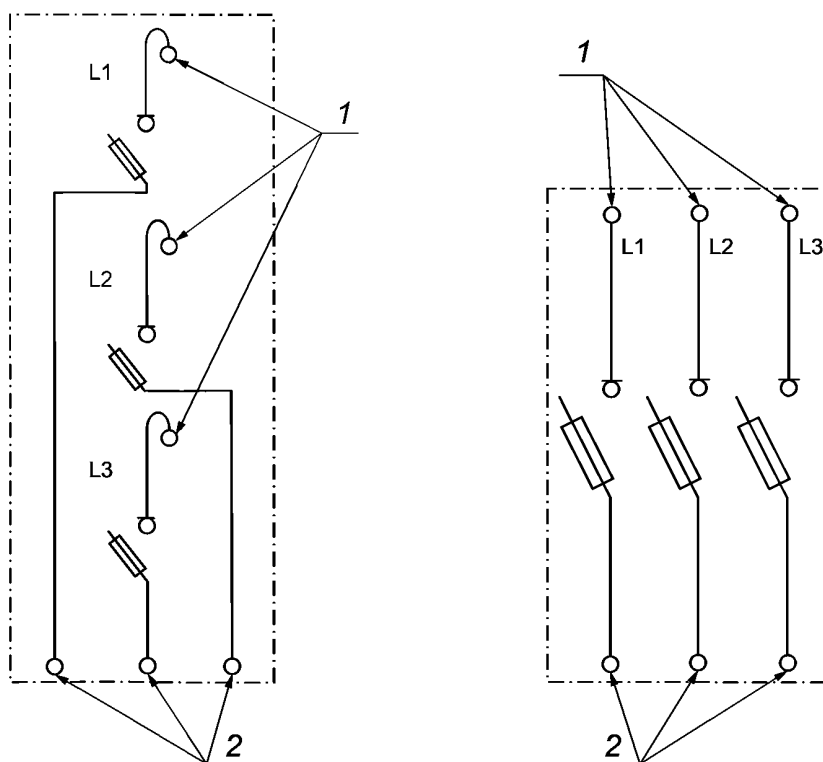
1 — выводы для шин; 2 — выводы для кабелей
