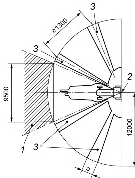
б) Полукруг обзора вперед по 5.3
