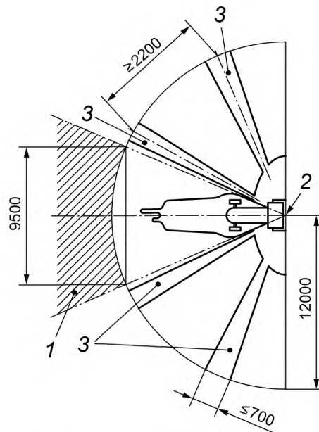
а) Полукруг обзора вперед по 5.1
