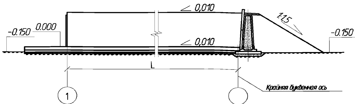
Рисунок 2 — Продольный разрез 1-1 наземного типа тупиковой сблокированной траншеи, состоящей из двух расположенных рядом траншей
