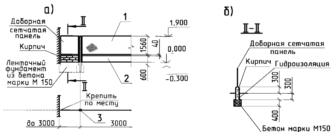
а) узел примыкания панели к стене; б) разрез II-II 1 — металлическая панель ограждения; 2 — железобетонная цокольная панель; 3 — железобетонная стойка
