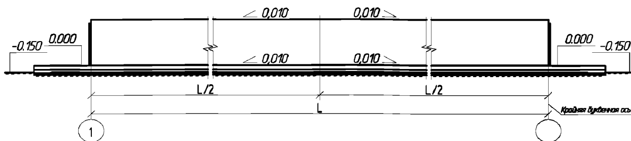
Рисунок 4 — Продольный разрез 1-1 проездной траншеи наземного типа
