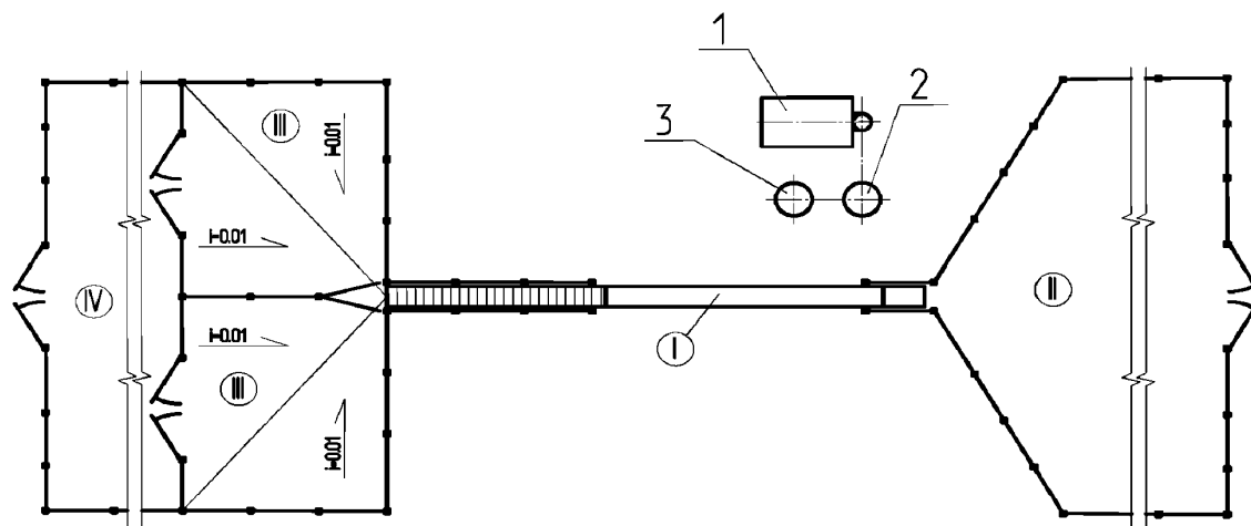
I — купочная ванна; II — накопительный загон с расколом; III — отжимная площадка; IV — площадка для обработанных животных. 1 — паровой котел; 2 — бак приготовления маточного раствора; 3 — бочка для креолина
