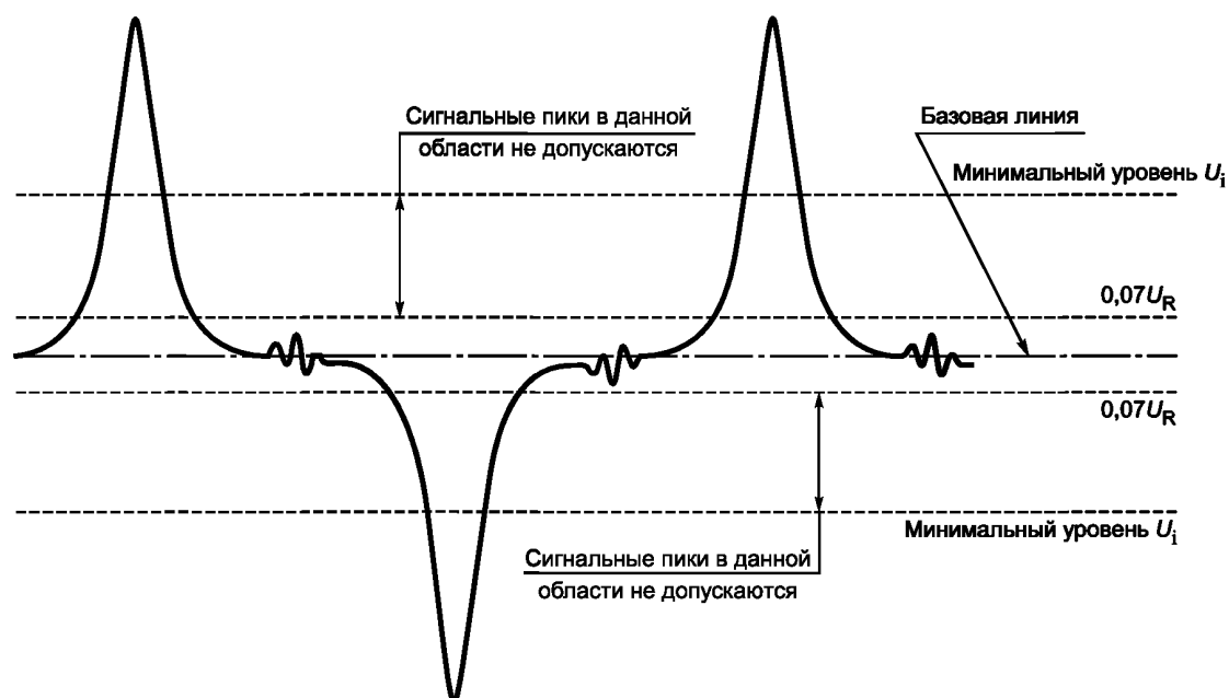
Рисунок 9 — Присутствие нежелательных пиков в форме сигнала
