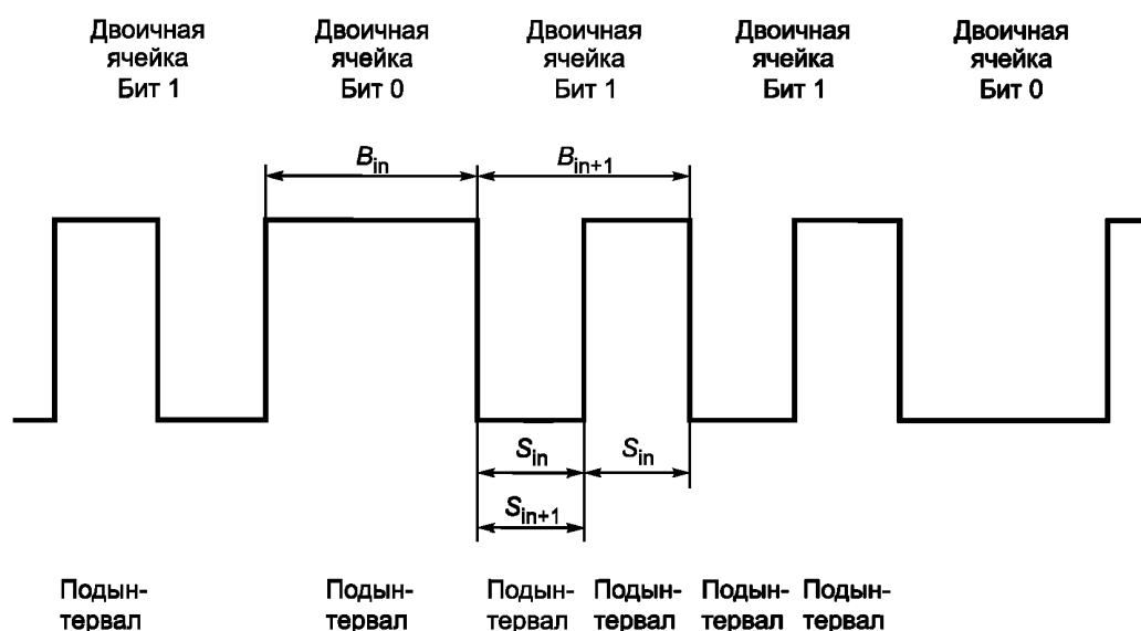
Рисунок 10 — Изменение промежутка между переходами потока
