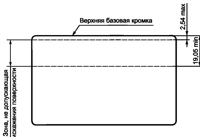
Рисунок — Зона на карте с магнитной полосой, где не допускаются искажения поверхности
