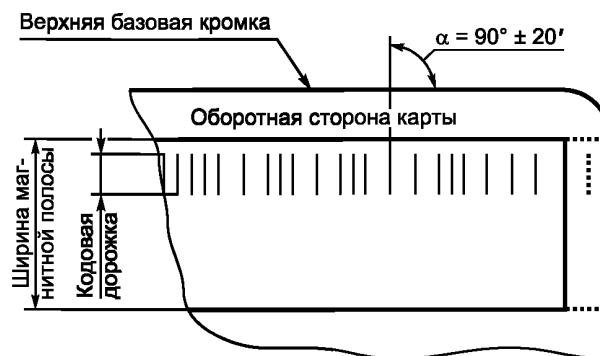
Рисунок 8 — Угол записи
