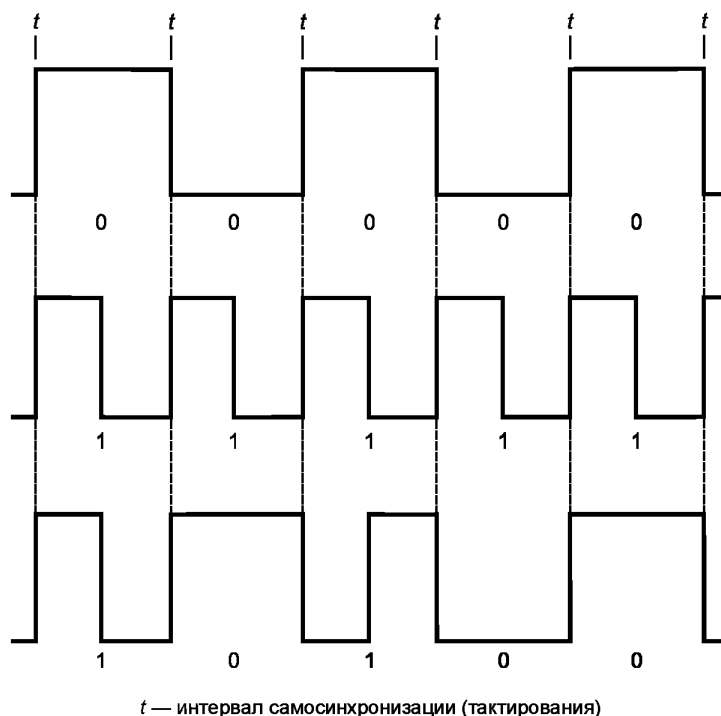
Рисунок 7 — Пример двухчастотного синфазного кодирования
