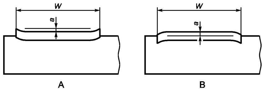
Рисунок 3 — Профиль поверхности
