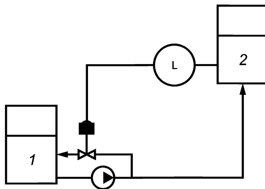
Рисунок В.5 — Технологическая схема для таблицы В.2
