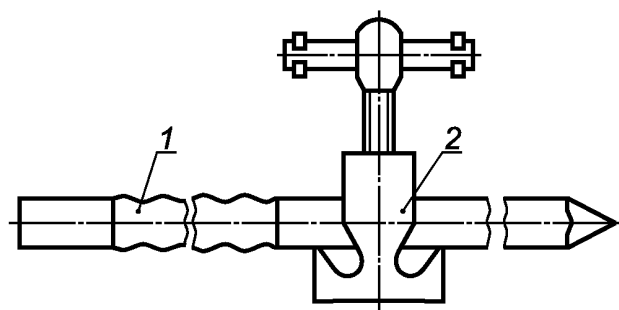
1 — стержень; 2 — зажим
