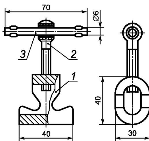
1 — зажим; 2 — болт М8х45 по ГОСТ 3033; 3 — вороток
