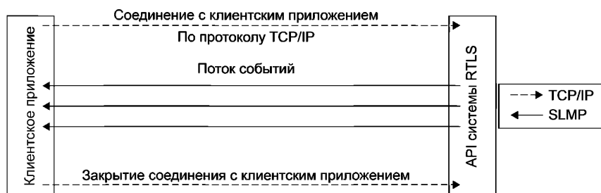
Рисунок 1 — Архитектура протокола SLMP
