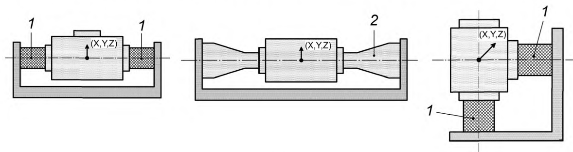
Рисунок 7 — Монтаж компонентов на вибростенде
