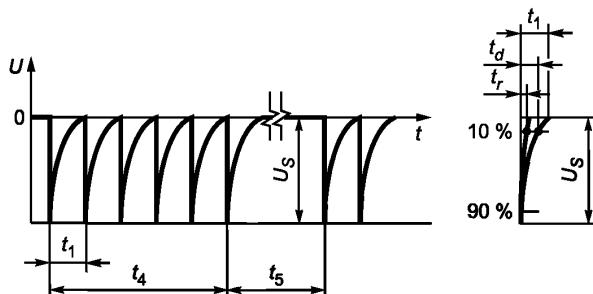
Рисунок 16 — Форма и параметры испытательных импульсов 3а
