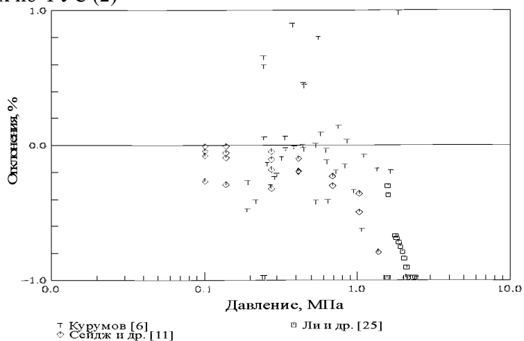
Рис. Б5. Отклонения экспериментальных p, v, T -данных в газовой фазе от рассчитанных по ФУС (2)
