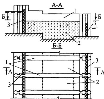
1 – бетон I очереди; 2 – бетон II очереди, уложенный под защитой затворов; 3 – затворы (шандоры)
