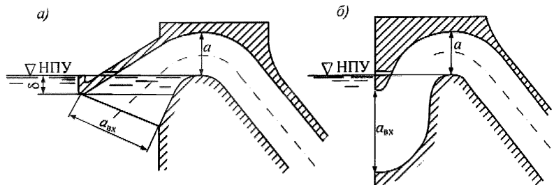
Рисунок 31 – Типы сифонных водосбросов в теле бетонных плотин (а) и в теле грунтовой плотины (б)
