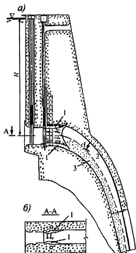
1 – зона отрыва потока за дефлекторами, установленными перед пазом основного плоского затвора; 2 – основной сбросной поток воды по вогнутому потолку; 3 – зона, заполненная воздушно-водной смесью или воздухом
