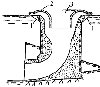
1 – входные отверстия; 2 – капор; 3 – отверстия для сброса мусора
