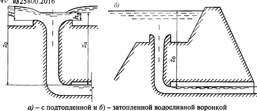
Рисунок 24 – Схемы гидравлических условий работы шахтных водосбросов
