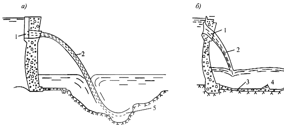
1 – глубинный водосброс; 2 – отброшенная струя; 3 – бетонное крепление; 4 – гаситель; 5 – воронка размыва
