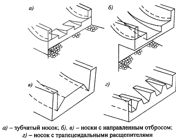
Рисунок – 38 Различные типы носков-трамплинов
