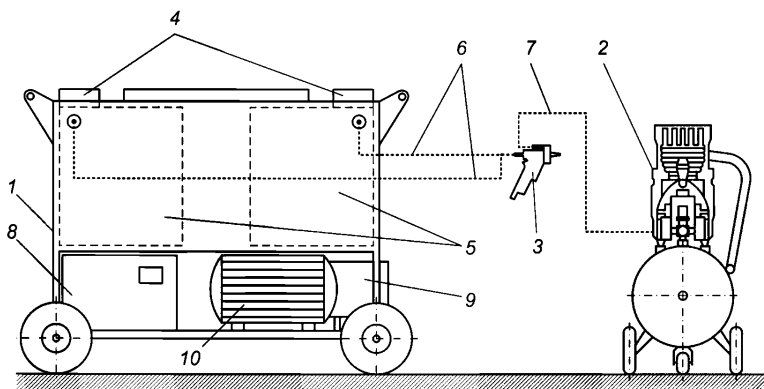
1 – установка для нанесения полиуретанового вяжущего; 2 – компрессорная станция; 3 – пистолет-распылитель; 4 – заливочная горловина; 5 – емкость для компонента; 6 – шланг подачи компонента; 7 – шланг подачи воздуха; 8 – системы дозирования и термостатирования; 9 – система насосов для подачи компонентов; 10 – приводные двигатели
