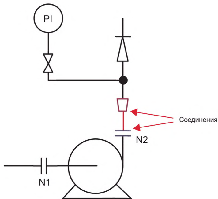
Рисунок 2 — Связь схематических элементов
