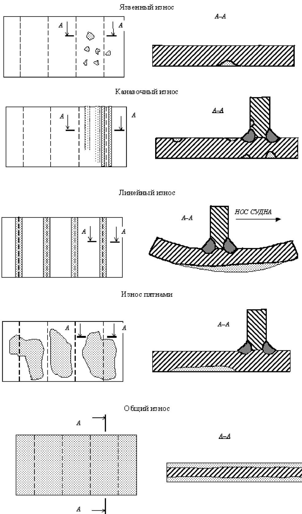
Рис. 1.2.1-2 Виды износов
