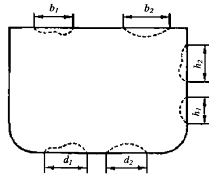
Рис. 3.3.2.1 Вмятины
