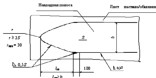
Рис. 5.2.1.5-2 Оформление окончаний накладных полос
