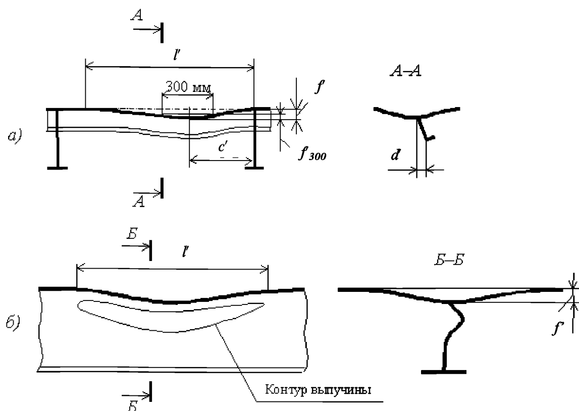
Рис 3.3.4.2 Измерение параметров выпуклин: а — для балок основного набора; б — для балок рамного набора и листовых элементов
