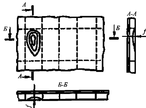
Рис. 3.3.2.4-2 Бухтина
