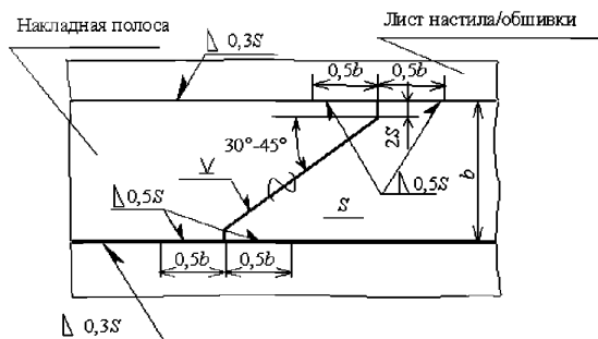
Рис. 5.2.1.5-1 Оформление стыков накладных полос
