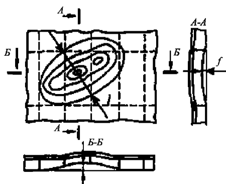
Рис. 3.3.2.4-3 Вмятина
