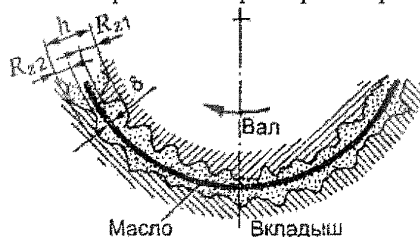
Рис.3 Масляный слой при установившемся режиме работы
