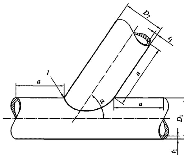
Рис. 8.2.2.7 Проба узла сочленения труб:
