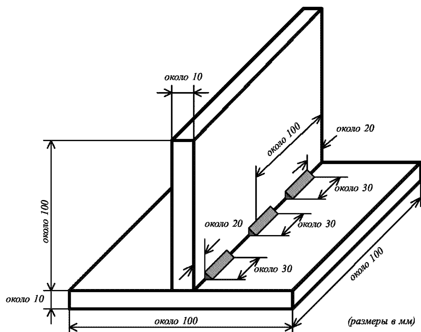
Рис. 10 Тавровая проба для сварки сборочных прихваток P_{2tack}
