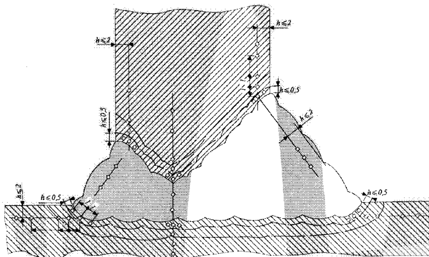
Рис. 6.4.4.5-4 Схема расположения точек замера твердости в тавровых соединениях со сплошным проваром
