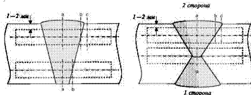
Рис. 6.4.4.4-2 Схема вырезки и расположения надреза на образцах для испытаний на ударный изгиб для технологических процессов сварки с погонной энергией \leq 50 кДж/см: а — надрез по центру шва (WM); б — надрез по линии сплавления (FL); с — надрез по ЗТВ на расстоянии 2 мм от линии сплавления (FL + 2)
