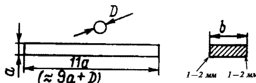
Рис. 6.4.4.2-1 Образцы для испытаний на статический изгиб:
