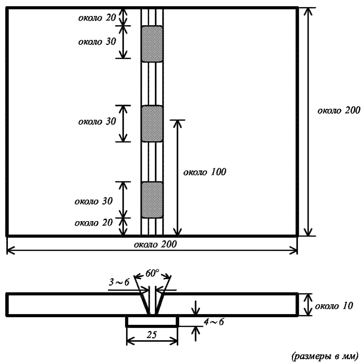
Рис. 9 Стыковая проба для сварки сборочных прихваток P_{1tack}
