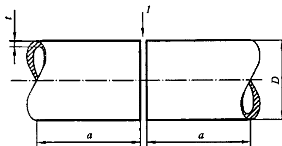
Рис. 8.2.2.5 Проба стыкового соединения труб: I — конструктивные элементы подготовки кромок и зазор в соответствии с пСПС; t — толщина основного металла; a \geq 150 мм; D — наружный диаметр трубы
