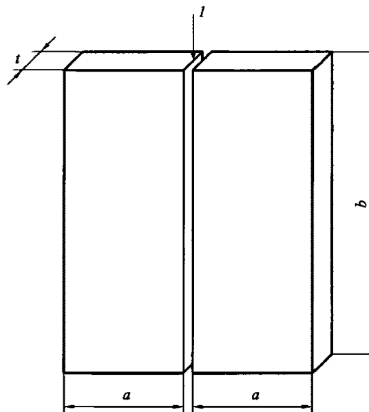
Рис. 8.2.2.4 Проба стыкового соединения листов: I — конструктивные элементы подготовки кромок и зазор в соответствии с пСПС; t — толщина основного металла; a \geq 150 мм (размер образцов на статический изгиб может потребовать увеличения); b \geq 350 мм
