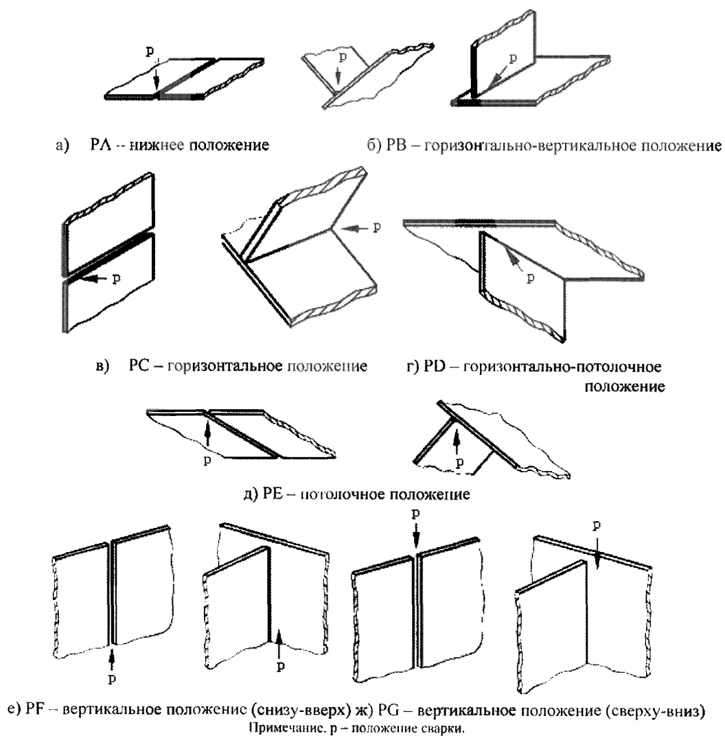
Рис. 1 Положения при сварке пластин».
