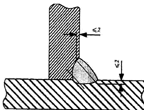
Рис. 6.4.4.5-5 Схема расположения линий замера твердости в тавровых соединениях без разделки кромок, выполненных угловым швом
