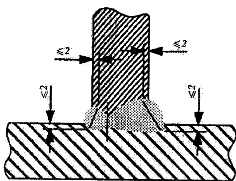
Рис. 6.4.4.5-3 Схема расположения линий замера твердости в тавровых соединениях со сплошным проваром
