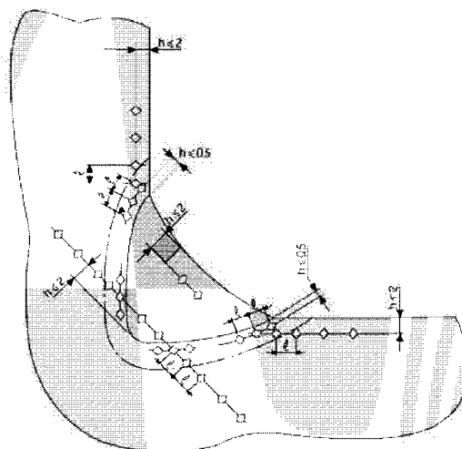
Рис. 6.4.4.5-6 Схема расположения точек замера твердости в тавровых соединениях без разделки кромок, выполненных угловым швом
