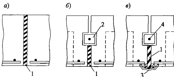
а – шов, заполненный шнуровым асбестом; б – то же, с бетонным брусом; в – то же, с металлическим компенсатором; 1 – шнуровый асбест, смоченный в глиняном растворе; 2 – бетонный брус; 3 – компенсатор; 4 – стальной стержень диаметром 6 мм
