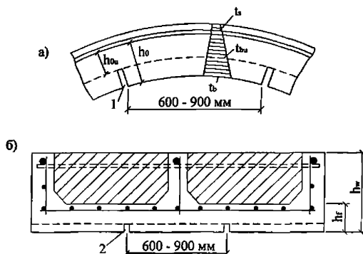
Рисунок 9.5 – Швы со стороны нагреваемой поверхности в конструкциях из жаростойкого бетона
