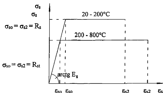
Рисунок 5.2 - Расчетная двухлинейная диаграмма растянутой арматуры
