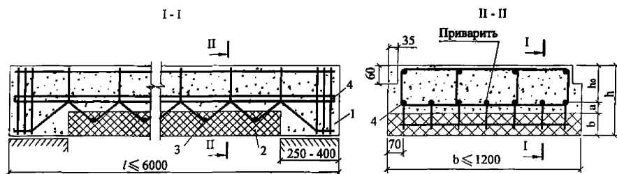
Рисунок 9.6 – Конструкция изгибаемого железобетонного элемента, нагреваемого до температуры более 400 °С со стороны растянутой зоны
