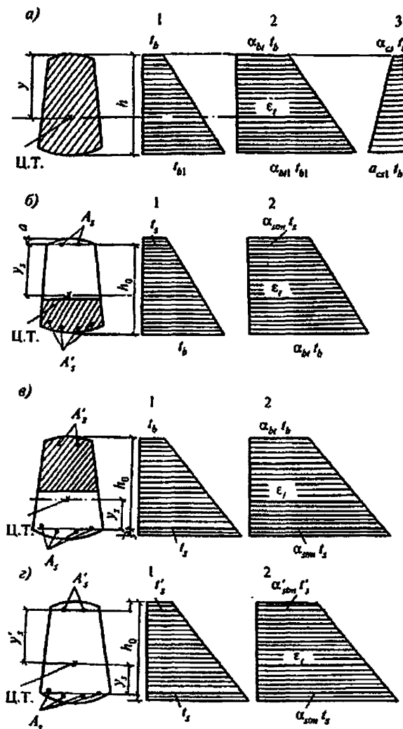
а – бетонного и железобетонного элемента без трещин; б – железобетонного элемента с трещинами в растянутой зоне, расположенными у менее нагретой грани; в – то же, у более нагретой грани; г – железобетонного элемента с трещинами по всей высоте сечения; Ц.Т. – центр тяжести приведенного сечения
