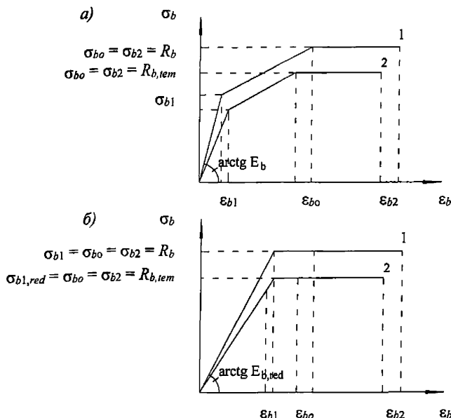
Рисунок 5.1 – Расчетные диаграммы состояния сжатого бетона
