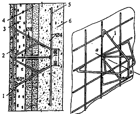
Рисунок 9.8 – Пространственный анкер в многослойной конструкции панели с железобетонной несущей плитой
