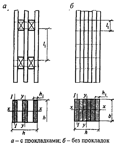
Рисунок 2 – Составные элементы
