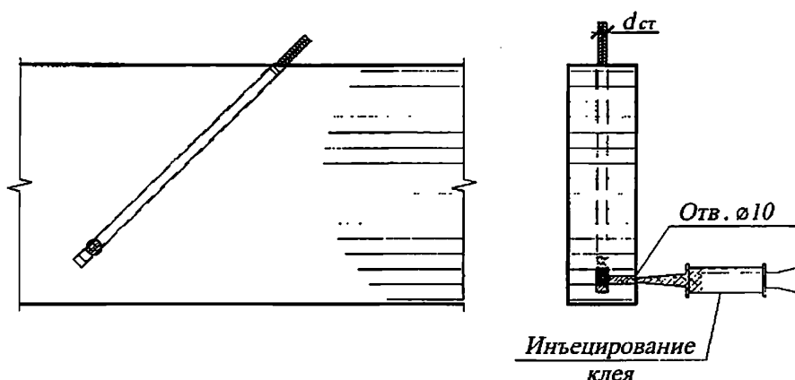
Рисунок Ж.2 – Схема подачи клея под давлением
