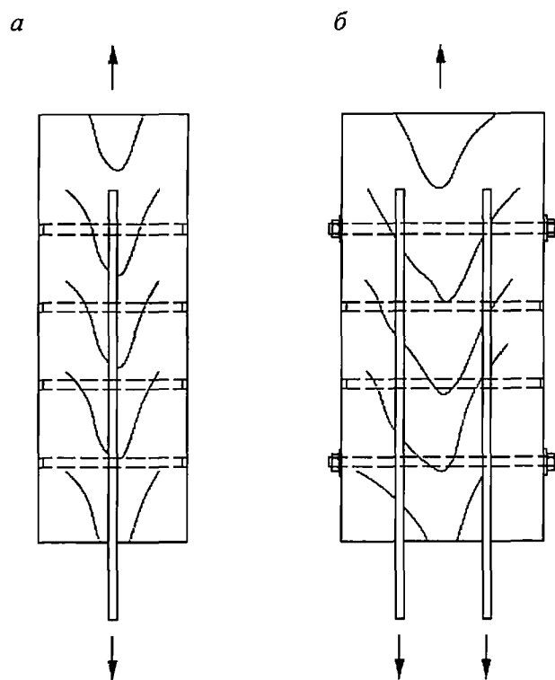
Рисунок 11 – Нагельные соединения с накладками
