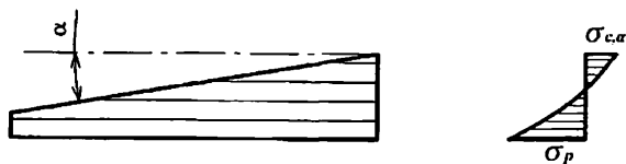
Рисунок 23 – Односкатная балка
