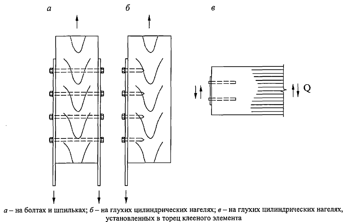
Рисунок 11 – Нагельные соединения с накладками
