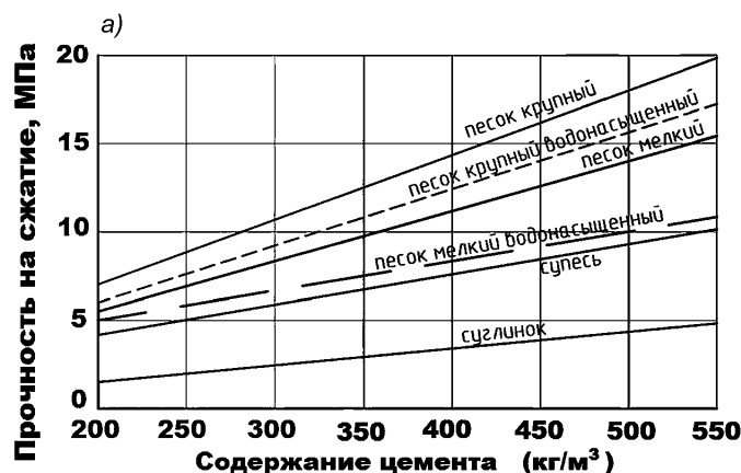
Рисунок 6.1, лист 1 — Зависимость расхода цемента для обеспечения прочности грунтоцемента различных видов грунтов
