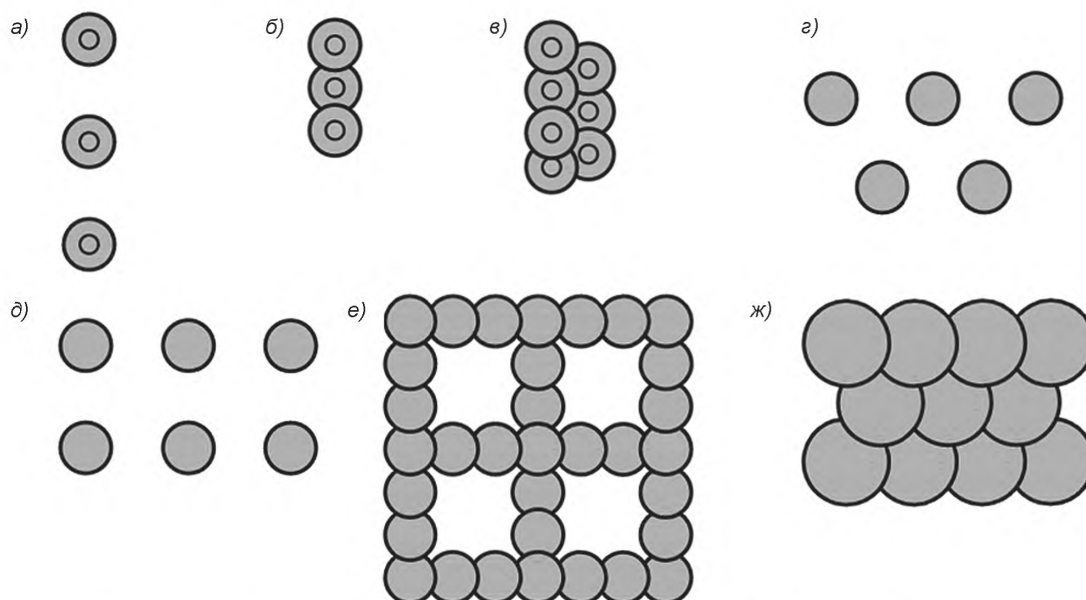
а) — одиночно; б) — в один ряд; в) — в два ряда; г) — по треугольной сетке; д) — по квадратной сетке; е) — в виде ячеистой структуры; ж) — сплошным массивом
