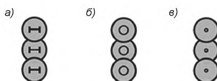
а) — двутавром; б) — трубой; в) — тремя буроими штангами с накатанной винтовой поверхностью
