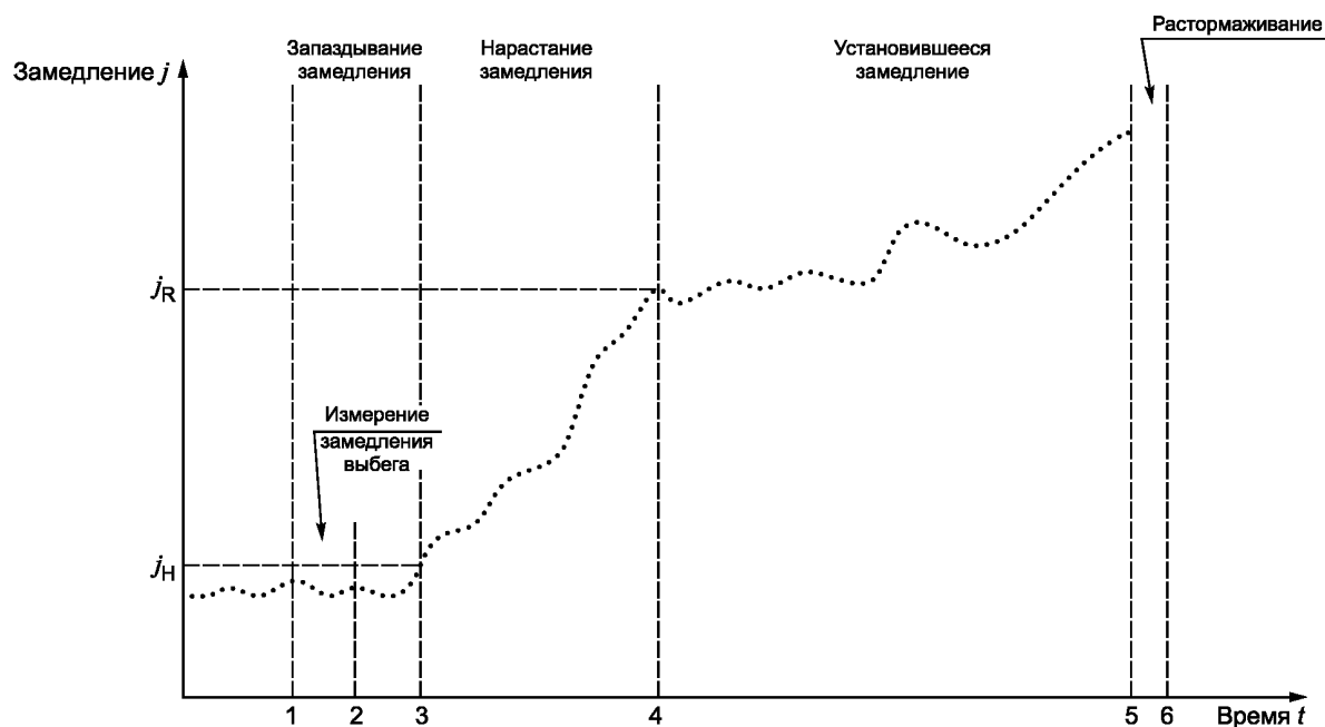
В.1 Схематический график замедления КТС (тормозная диаграмма) при торможении в дорожных условиях
