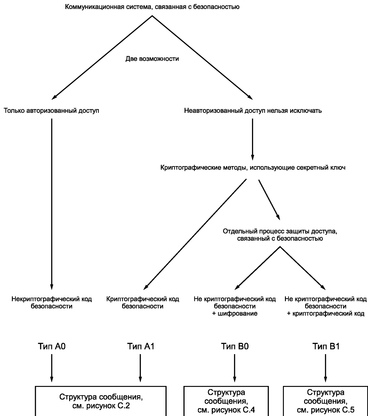
Рисунок С.1 — Классификация связанных с безопасностью систем связи
