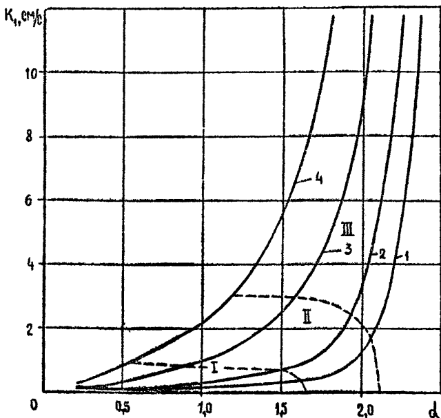
Рис. I. Изменение водопроницаемости проволочного фильтра диаметром 100 мм в зависимости от K_2 гравийной обсыпки:
