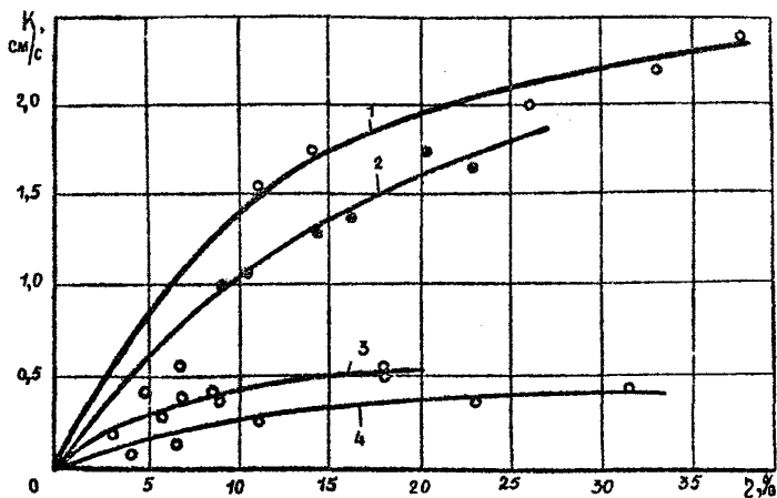
Рис. 9. Водопроницаемость фильтров различных типов в зависимости от скважности:
