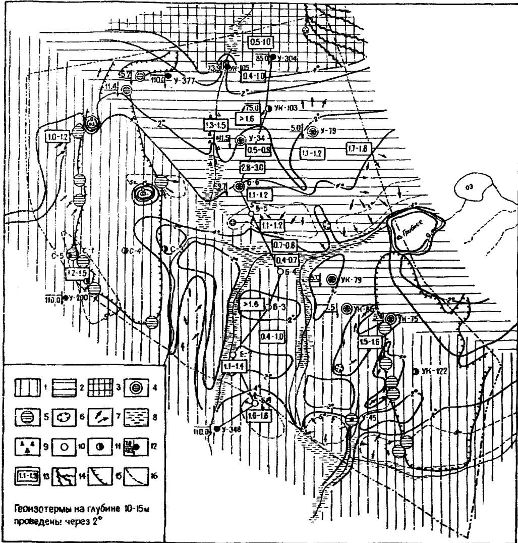
Рис.3. Инженерно-геоклиматическая карта месторождения полезных ископаемых на Крайнем Севере Сибири; намечается разработка открытым способом
