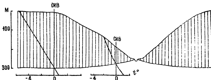
Рис.5. Максимальное распространение (заштриховано) и минимальная температура толщи мерзлых пород на Крайнем Севере свойственны водораздельным участкам, талики - долинам и озерным впадинам
