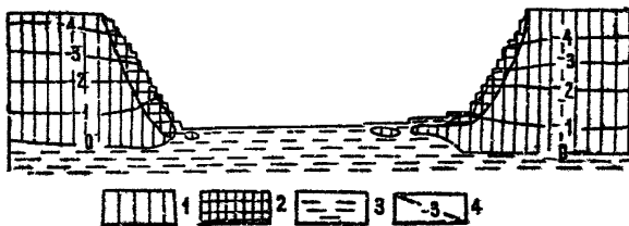
Рис.9. Инженерно-геокриологический профиль карьера, отрабатываемого в районе Крайнего Севера
