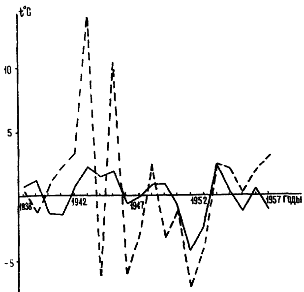
Рис.7. График средних годовых (сплошная линия) и сумма средних месячных температур воздуха (пунктир) за теплый сезон в Норильске за 20 лет (1938-1957). Координата времени занимает положения, соответствующие оси колебаний той и другой характеристики (многолетним средним значениям их: -8,9^{\circ}\text{C} и 36,3^{\circ}\text{C} ).
