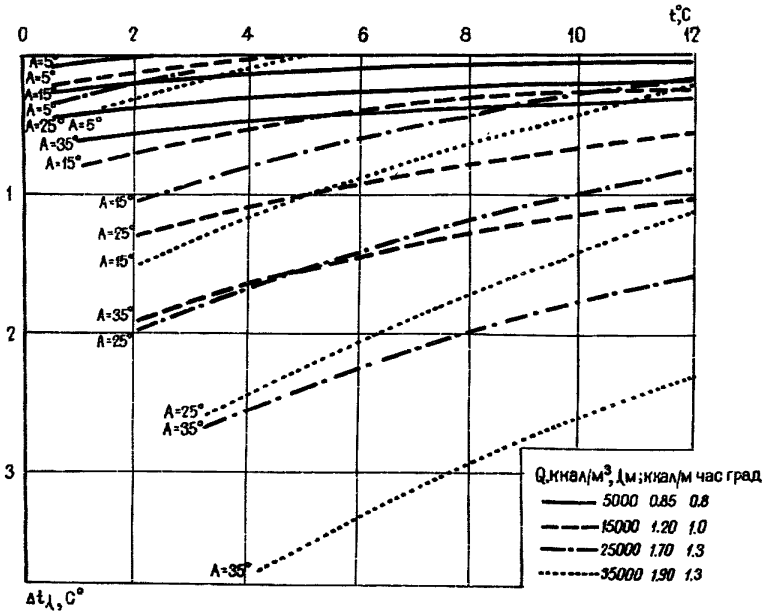
Рис.8. Номограмме для определения величины температурной сдвижки в слое сезонного протаявания (промерзания) пород
