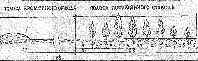
ТИП-IV-A насыпь при наличии снегозащитной полосы
