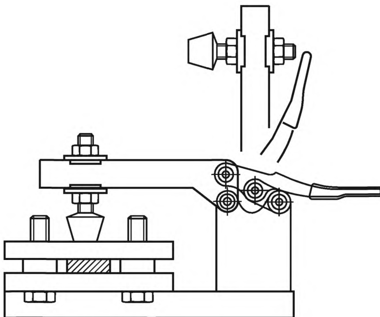
Рисунок 2 — Пример быстросъемного механизма
