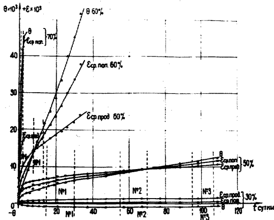
Рис. 4. Кривые ползучести образцов сильвинита, испытанных в лабораторных условиях.
